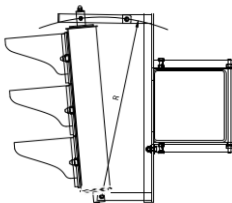
Schuifconstructie voor kokerbalkportaal t.b.v. 1, 2 en 3 lichter Afmeting 140 t/m 300 mm volgens opgave
