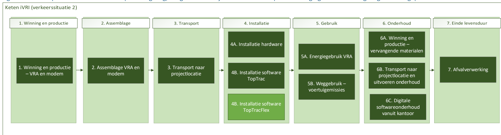
Figuur 6. Levenscyclus van een iVRI met TopTrac-regeling, aangevuld met bijkomende ketenstap ter toevoeging van de Flex-regeling zoals toegepast in verkeerssituatie 2.
